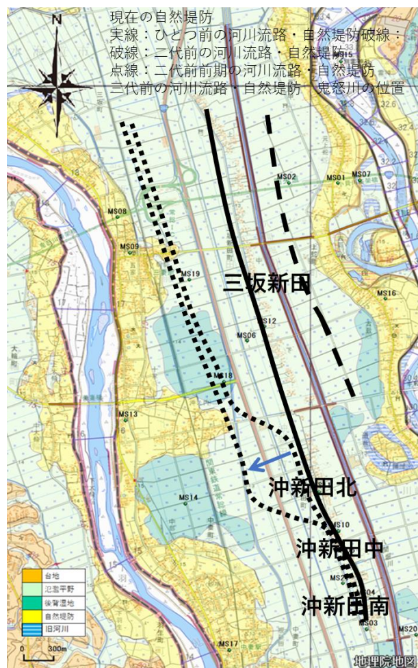
図2 河道変遷過程の推定結果(背景は治水地形分類図)
