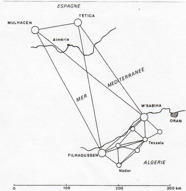
図 1 スペイン—アルジェリア渡海三角測量
